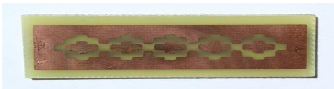
Figura 7 – Verso do filtro de microfita. Defeito DGS no plano terra.
