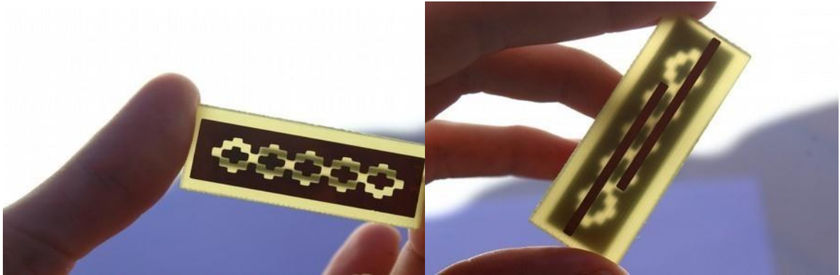
Figura 9 – Visualização das linhas de alimentação e do defeito DGS no plano terra.
