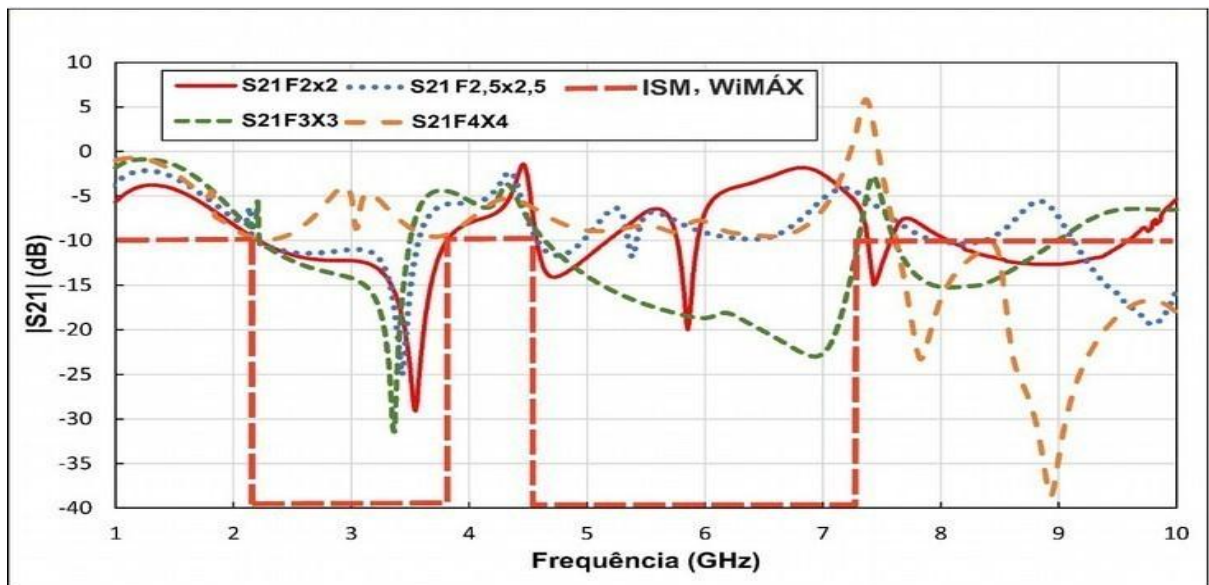
Gráfico 1 – Simulações do Ansoft Designer para os quatro filtros de microfita com defeitos DGS no plano terra.
