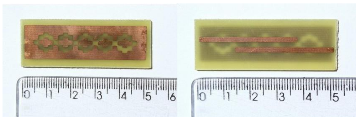
Figura 8 – Dimensional do filtro de microfita com defeitos periódicos quadráticos.
