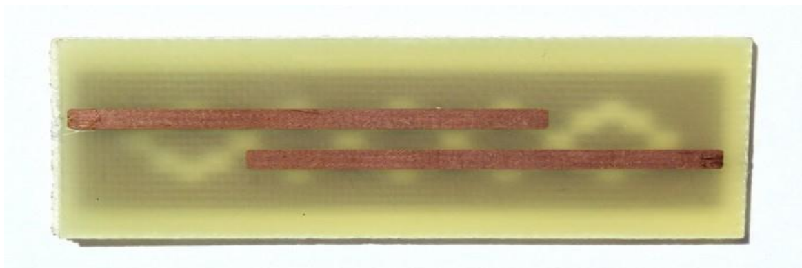
Figura 6 – Frente do filtro de microfita.
