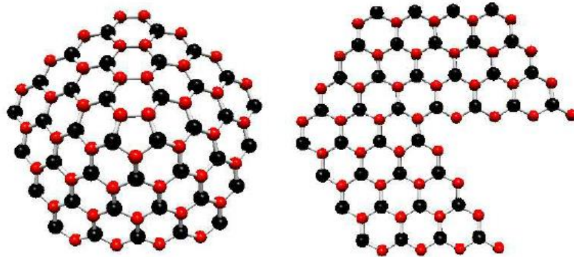
Figura 04 – Efeito de um setor removido de 60^\circ na folha de grafeno FONTE: Cortijo e Vezmediano, 2007 [CORTIJO, A.; VEZMEDIANO, M. 2007].
