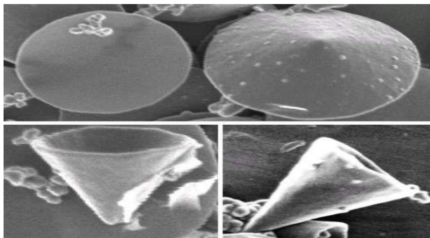
Figura 02 – Observação experimental de cones de grafeno. FONTE: Research Gate, 2019 [CARDENAS, S. 2014].
